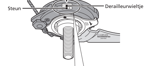
Steun
